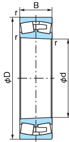
Коническое отверстие
