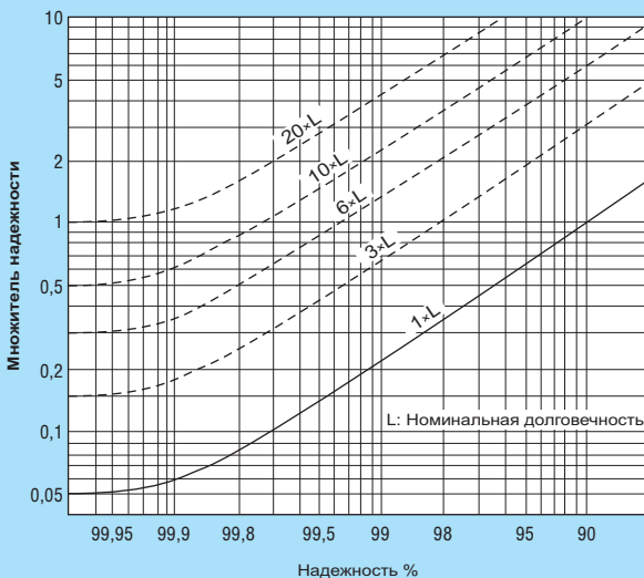
Рис 3.6 График надежности
