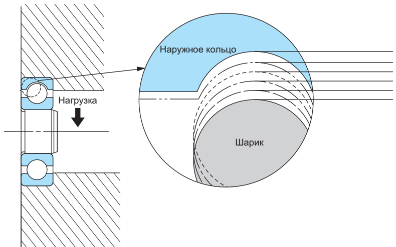
Рис. 8.3 Радиальный зазор подшипника
