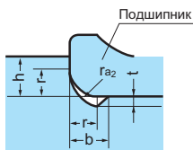
Рис. 8.8 Размеры фаски и радиус галтели
